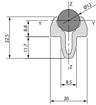
Profilo contemineto tondo Ø12 BPRGD0000020
