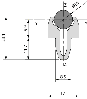
Profilo contemineto tondo Ø10 BPRGD0000032
