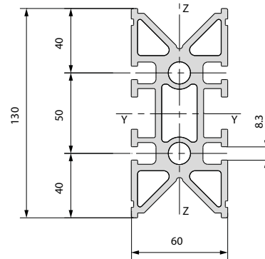
Profilo con guida a V 90° BPRGD0000025
