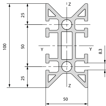
Profilo con guida a V 90° BPRGD0000023
