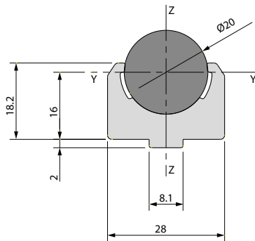
Profilo contemineto tondo Ø20 BPRGD0000021
