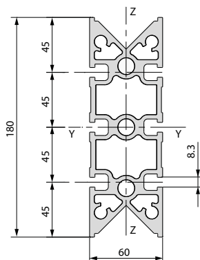
Profilo con guida a V 90° BPRGD0000026
