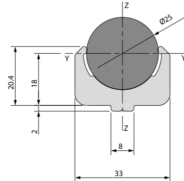
Profilo contemineto tondo Ø25 BPRGD0000022
